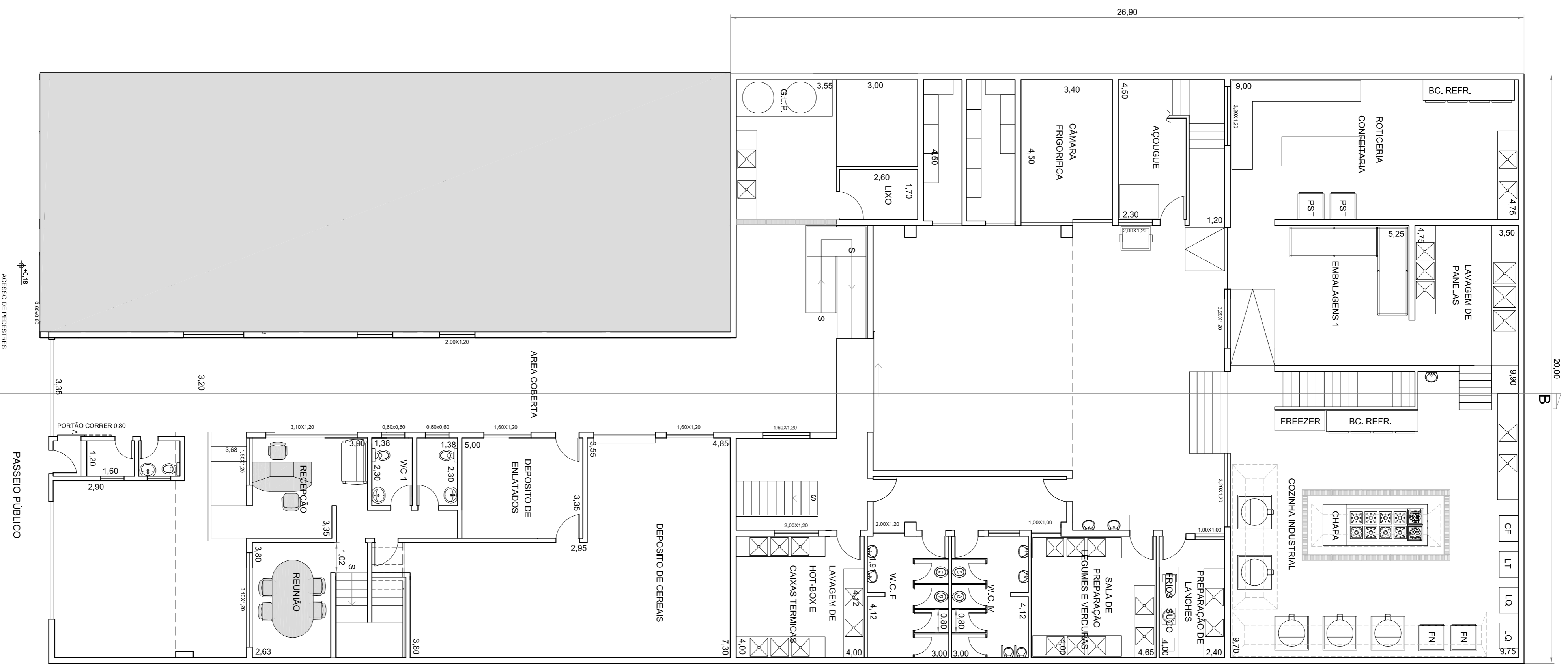
PLANTA - PAVIMENTO TÉRREO esc. 1:100
