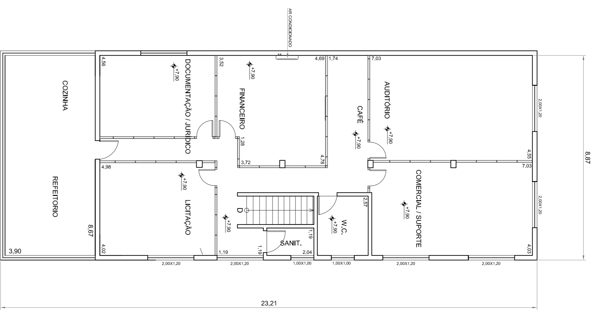
PLANTA - 2º ANDAR esc. 1:100
